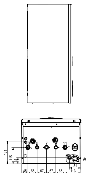
Vista inferiore
