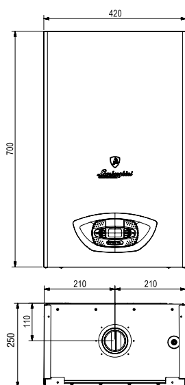
Vista superiore
